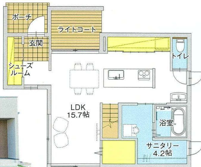
1階平面図
